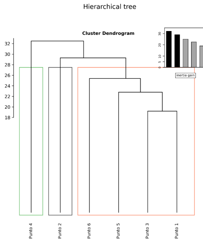
Figura 3. Análisis de clústers (dendrograma jerárquico) para los puntos de muestreo en el Humedal Bruselas Cananguchal, Florencia-Caquetá.
