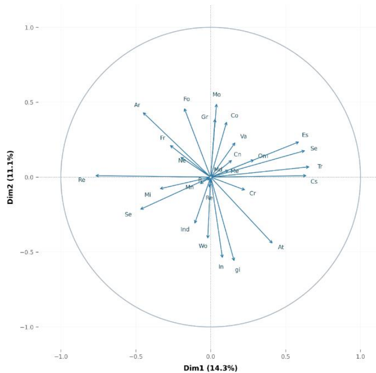
Figura 5. Círculo de correlaciones de los rasgos funcionales de las aves obtenido mediante Análisis de Componentes Principales (ACP) en el Humedal Bruselas Cananguchal, Florencia, Colombia.
