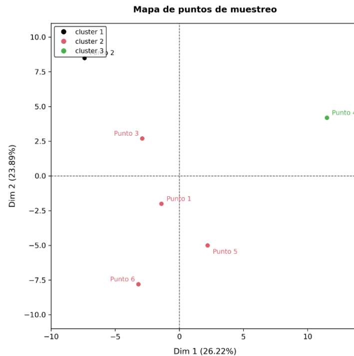
Figura 2. Análisis de Componentes Principales (PCA) para los puntos de muestreo en el Humedal Bruselas Cananguchal, Florencia-Caquetá.
