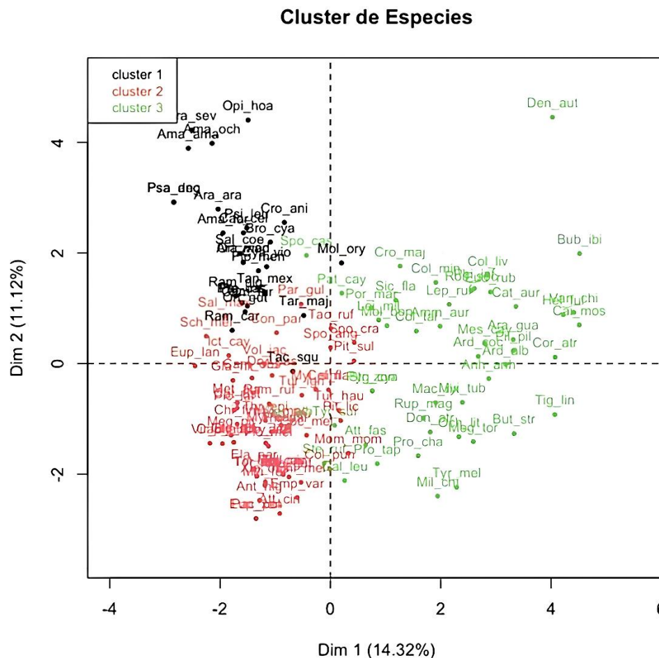
Figura 6. Análisis de Componentes Principales que muestra los agrupamientos (clústers) de especies de aves observadas en el Humedal Bruselas Cananguchal, Florencia, Colombia.
